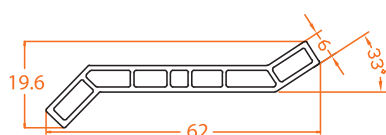
109.12 Louver
