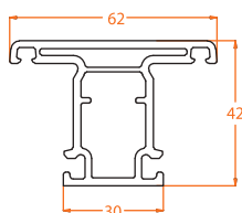
8804.1 Flush Door Mullion
