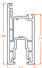
802.3 90mm Door Sash
