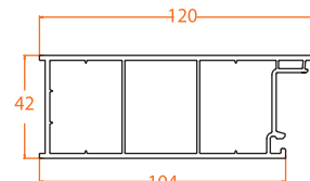
602.5 Flush Door Sash
