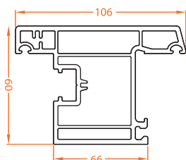
603.2 Outward Door Sash
