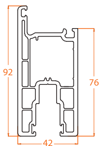
8802.3 92mm Door Sash
