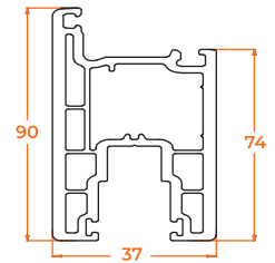
802.3 90mm Door Sash
