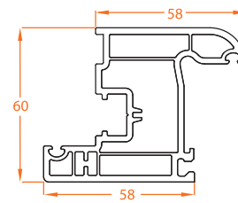
602.3 Inward Window Sash
