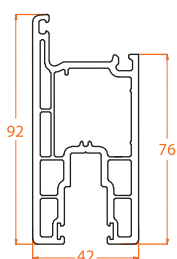
8802.3 92mm Door Sash
