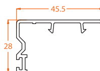
8807.1 Interlock
