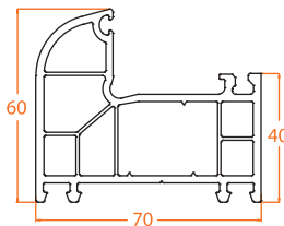
601.4 70/60 Frame
