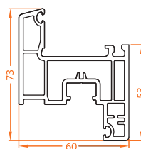
602.1 Inward Window Sash
