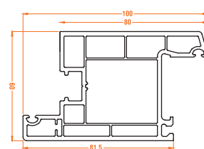
602.4 Inward Door Sash
