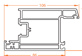
602.2 Inward Door Sash
