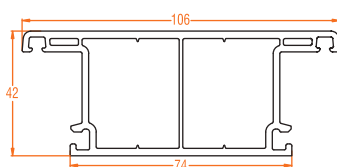
604.4 Flush Door Mullion
